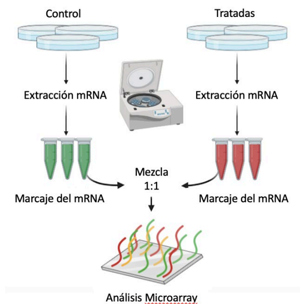
Figura 2. Esquema general de un experimento de transcriptómica.
