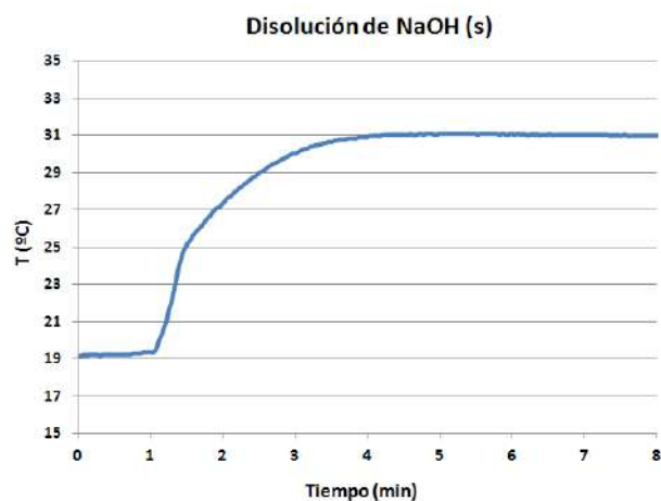
Figura 6. Curva obtenida tras la disolución de NaOH en agua. A partir de la diferencia de temperatura, y teniendo en cuenta la constante calorimétrica, se puede calcular la entalpía de disolución.
