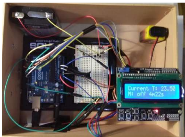
Figura 3. Microprocesador Arduino en el calorímetro electrónico.
