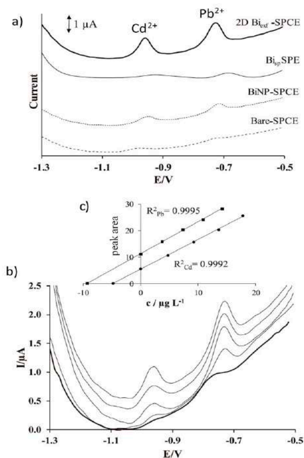
Figura 3: a) Voltamperogramas (nV.A) medidos en una disolución de 25 µg L -1 de Pb 2+ y Cd 2+ con electrodos serigrafados de carbono sin modificar (Bare-SPCE) y modificados con nanopartículas de Bi (BiNP-SPCE), Bi sputtered (Bi sp -SPCE) y bismuteno (2DBi exf -SPCE). b) y c)
